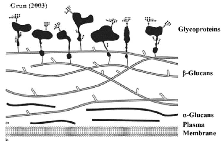
Zellwandbestandteile
